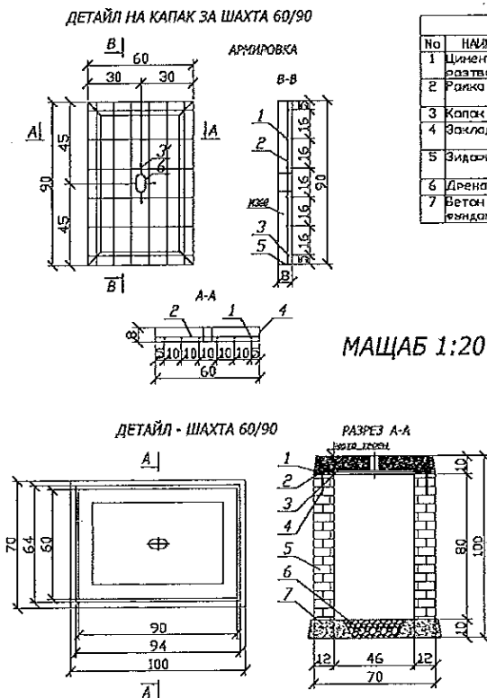
Фигура -. Кабелна шахта – единична
